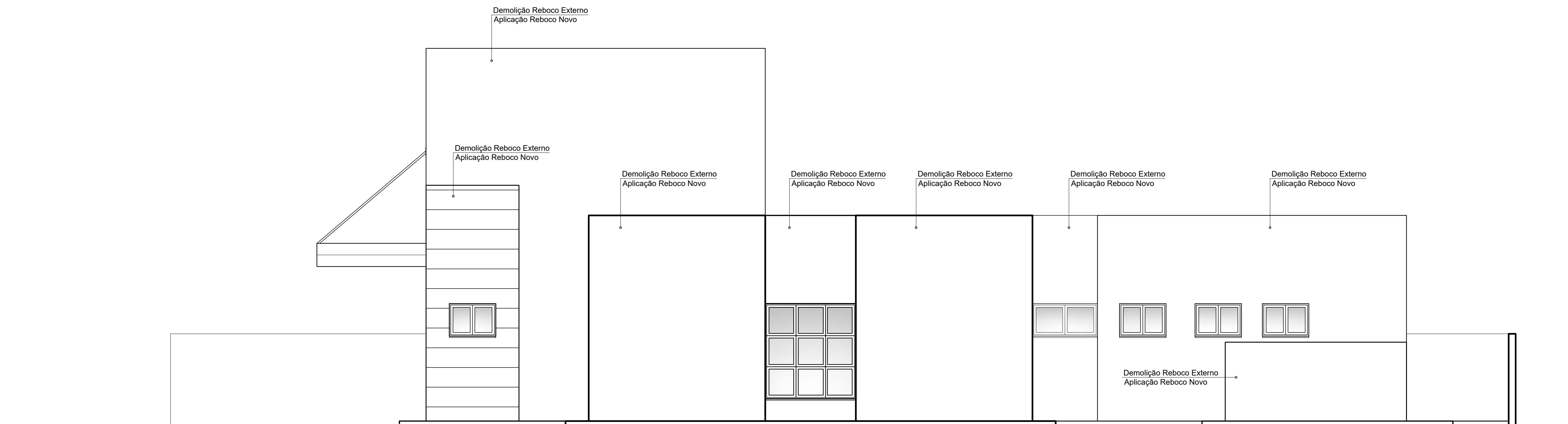
Fachada Lateral Esquerda (Oeste)
