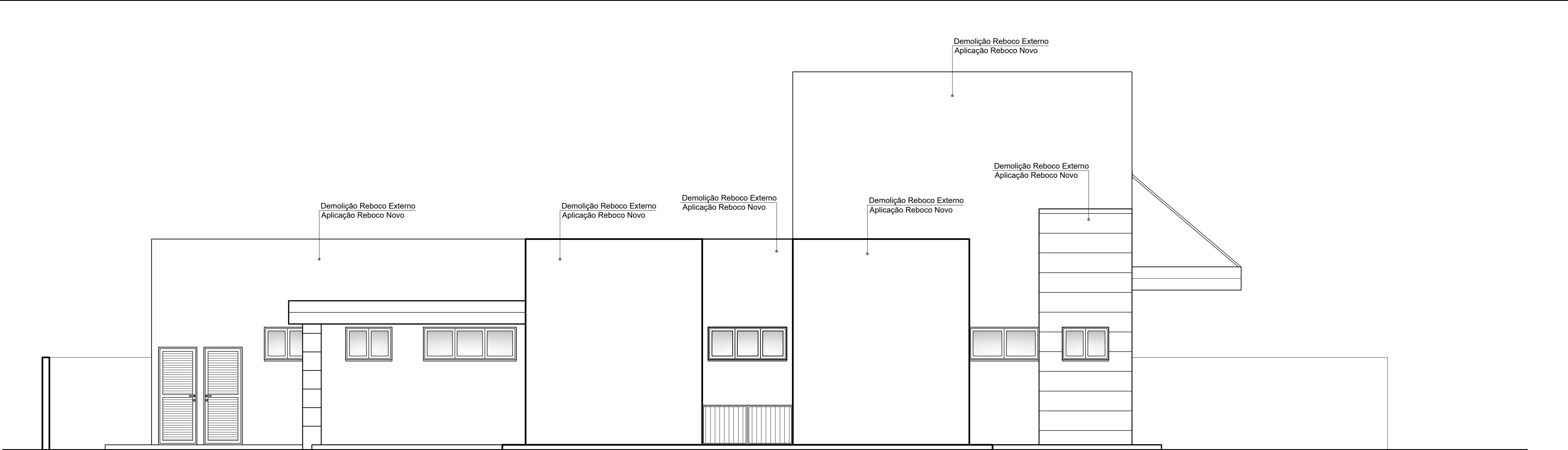
Fachada Lateral Direita (Leste)
