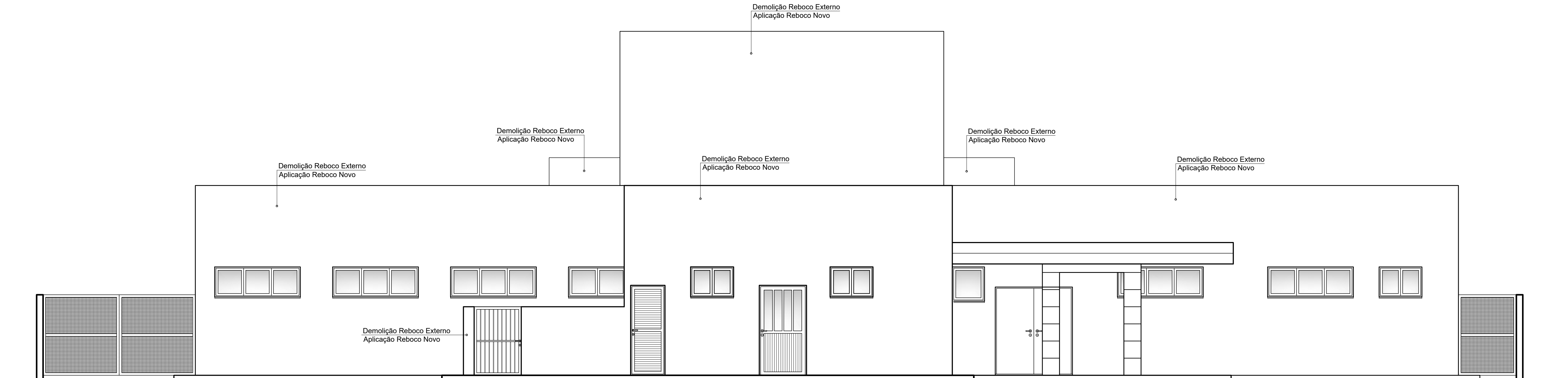
Fachada Fundos (Sul)
